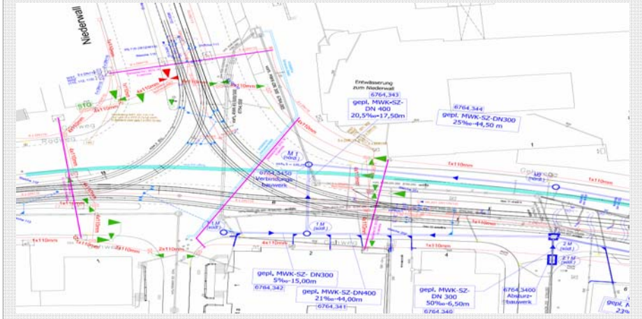
Umbau Detmolder Straße, Bielefeld | © STRABAG
