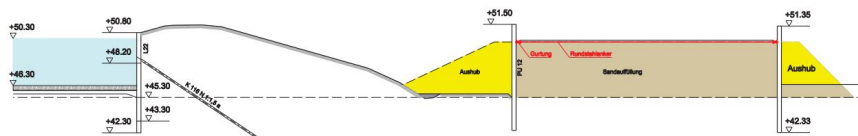
Bauphase II (Gurtung + Verankerung)
